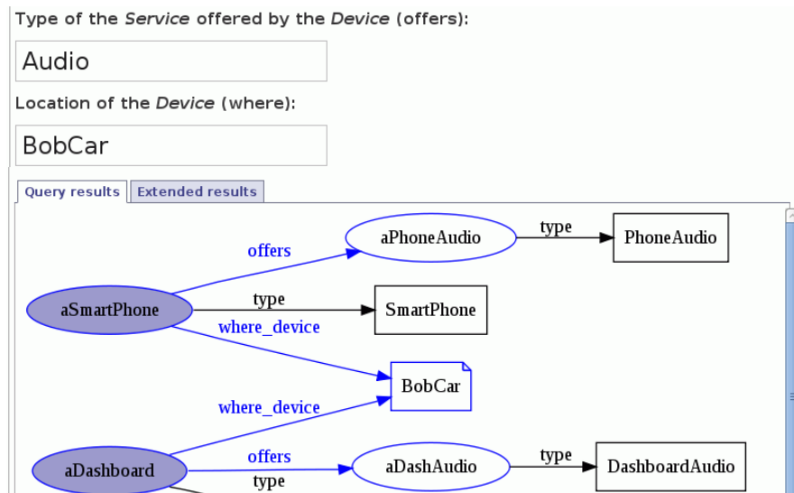
Figure 27. Exemple de Résultats de Requête.
