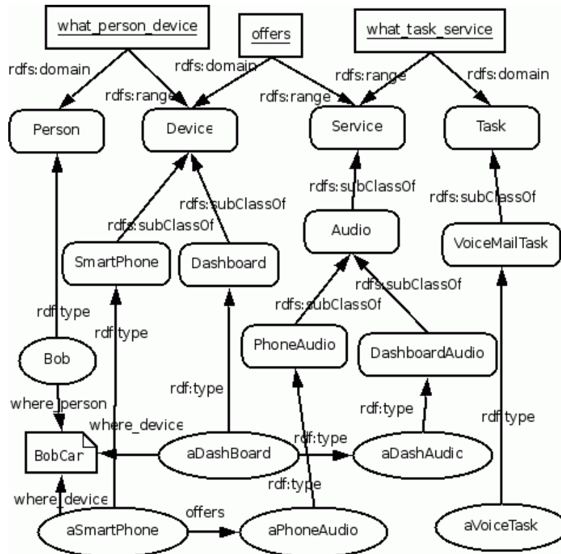
Figure 25. Exemple de modélisation d'un contexte.
