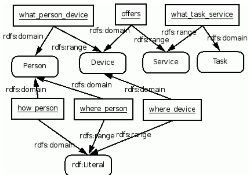
Figure 24. Métareprésentation du modèle de contexte en RDFS.
